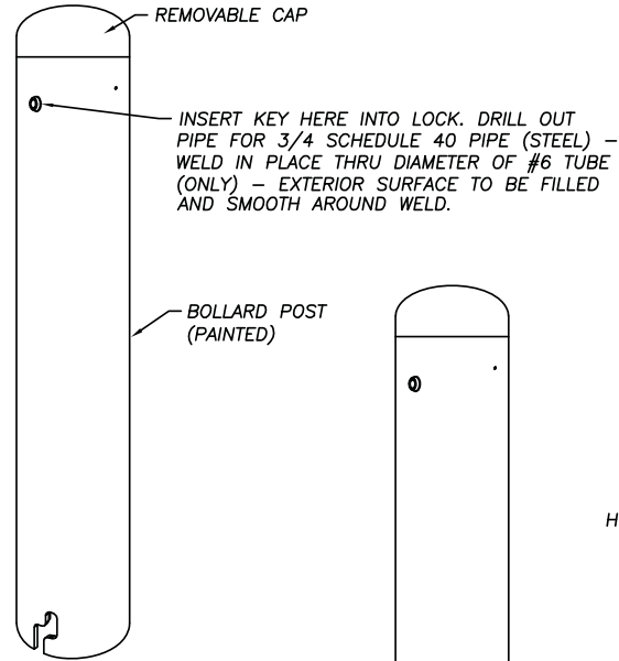
6.625" DIA. BOLLARD
