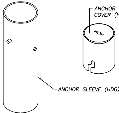
6.625" DIA. BOLLARD
