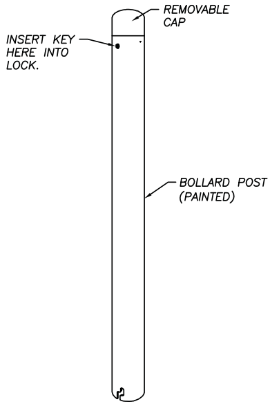
3" DIA. BOLLARD
